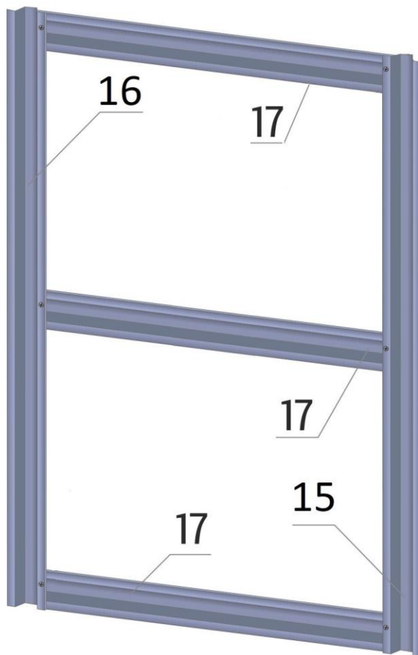
Obr. 6 – jedno křídlo dveří – celkem takto sestavte 4 křídla (pohled zvenku)
